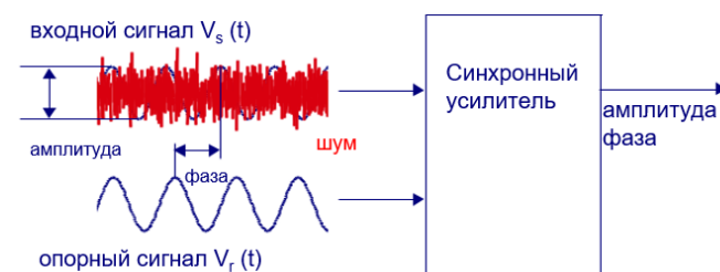
Рисунок 1. Синхронные усилители способны измерять амплитуду и фазу сигнала относительно определенного опорного сигнала, даже если сигнал полностью погружен в шум.
