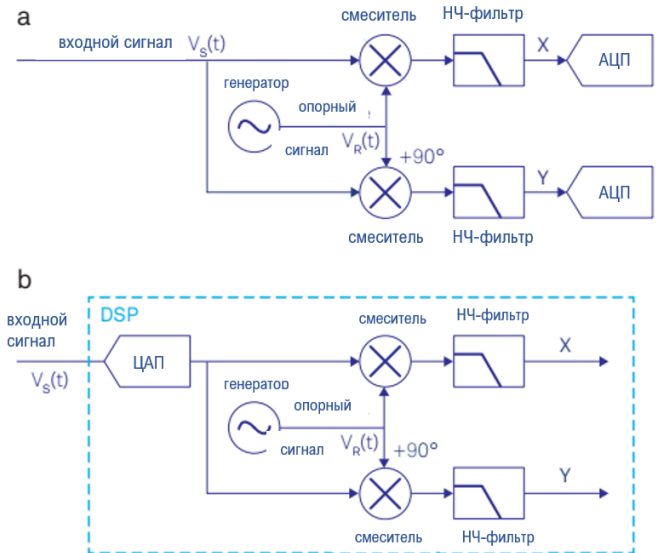
Рисунок 13. (а) Аналоговый синхронный усилитель: сигнал разделяется на два тракта, смешивается с опорным сигналом, фильтруется и затем преобразуется в цифровой. (б) Цифровой синхронный усилитель: сигнал оцифровывается, а затем умножается на опорный сигнал и фильтруется.
